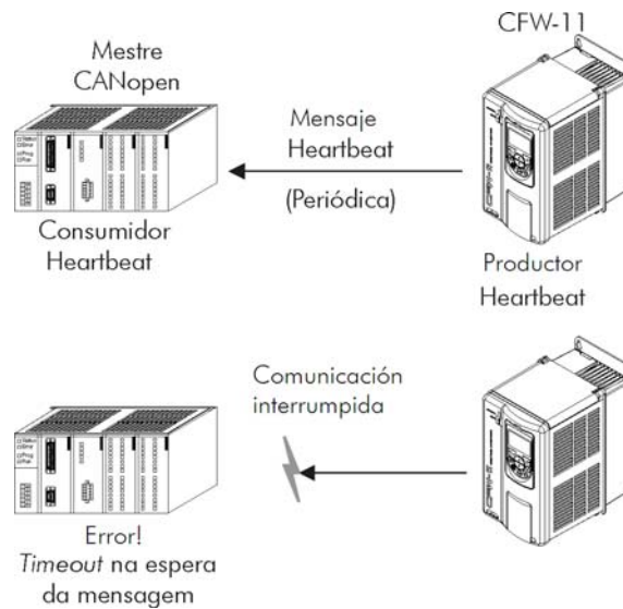
Figura 5-7 - Servicio de control de errores – Heartbeat
