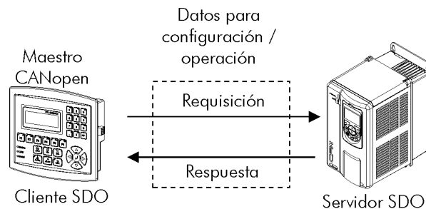
Figura 6.1: Comunicación entre cliente y servidor SDO
