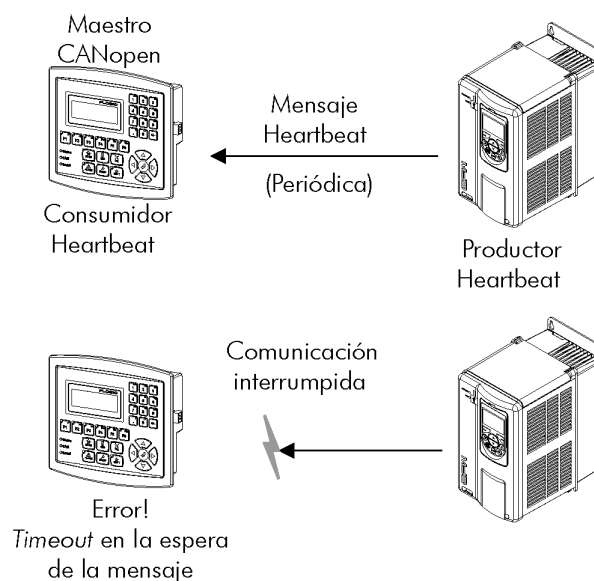
Figura 6.6: Servicio de control de errores – Heartbeat
