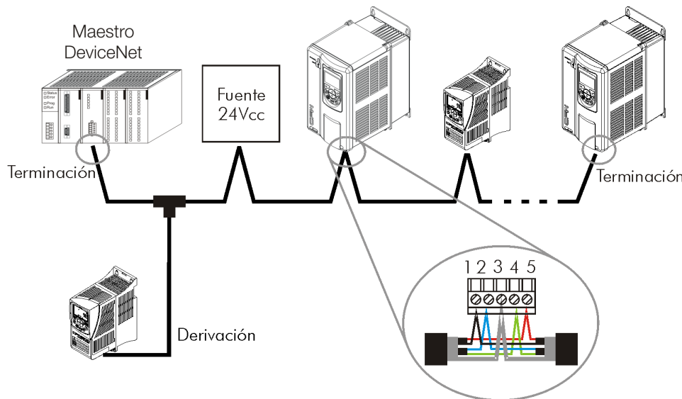
Figura 3.1: Ejemplo de instalación en red CANopen
