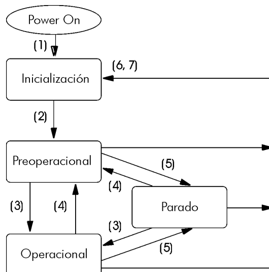
Figura 6.4: Diagrama de estados del nudo CANopen
