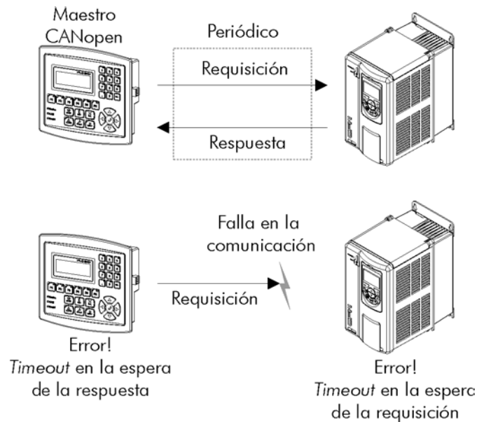
Figura 6.5: Servicio de control de errores – Node Guarding
