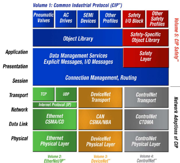
Figura 1.2: Estructura en capas del protocolo CIP
