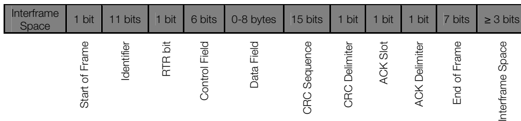
Figura 1.1: Frame de datos CAN
