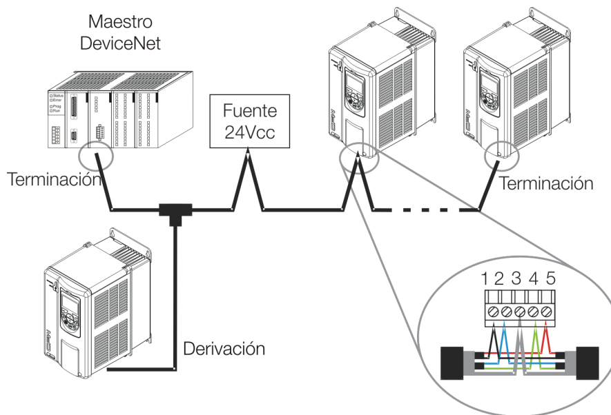
Figura 3.2: Ejemplo de instalación en red DeviceNet
