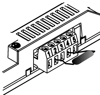
Figura 3.1: Ejemplo de instalación del resistor de terminación
